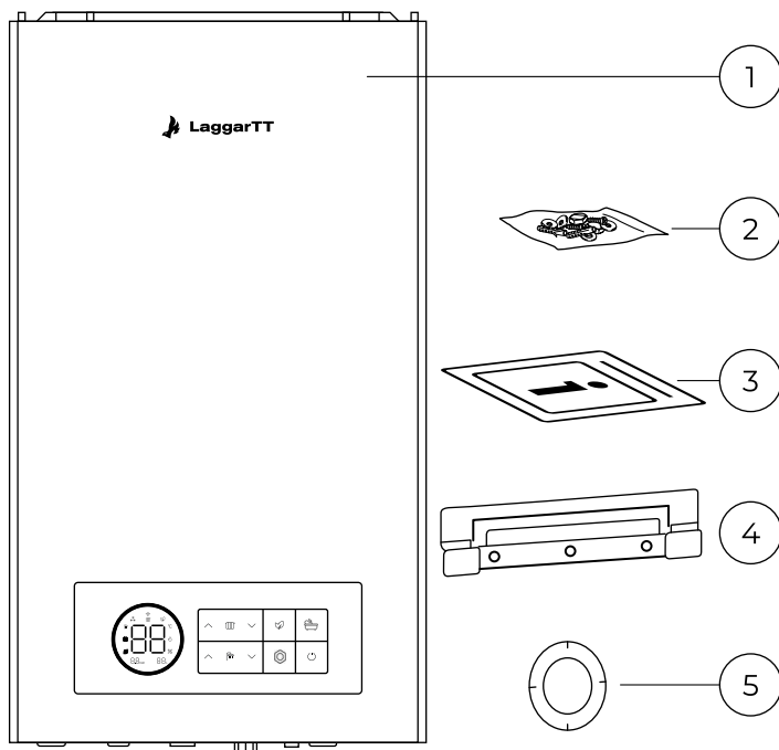
Рис. 1. Комплект поставки.
