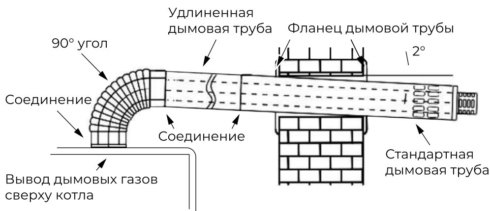
Рис.30. Пример монтажа схемы С12.
