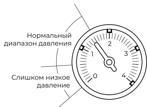
Рис. 8. Показания давления.
